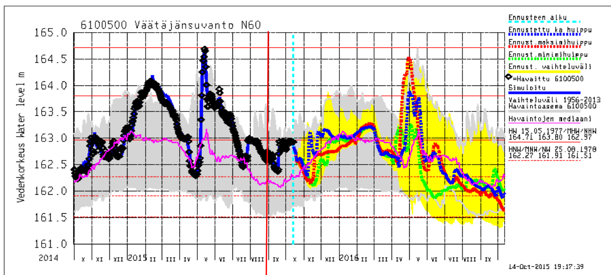
Kuva 1 Vedenkorkeus Väättäjänsuvanto
