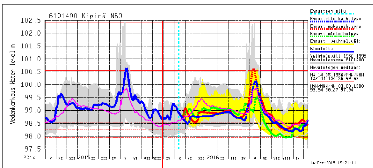
Kuva 2 Vedenkorkeus Kipinänkosket
